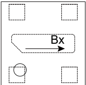
图 2-3 芯片敏感轴向图 (DFN4L 俯视图)
