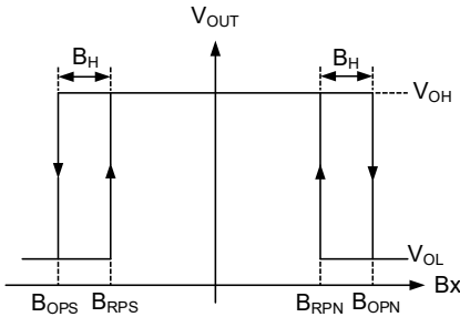
图 3 芯片磁场响应曲线
