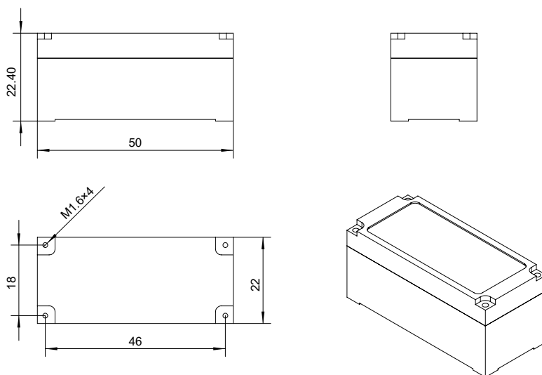
图 15 外形尺寸图 (尺寸单位: mm)
