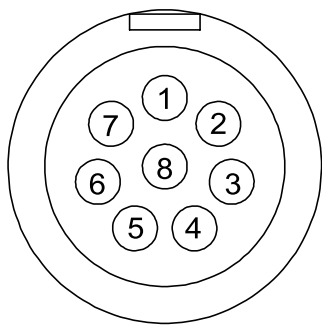
图 14 引脚定义
