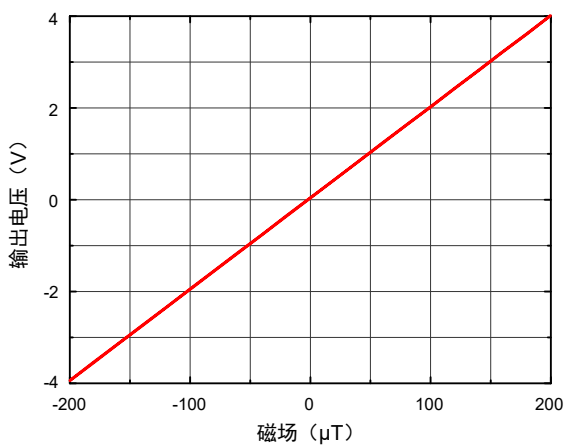
图 7 典型 VH 传输特性曲线
