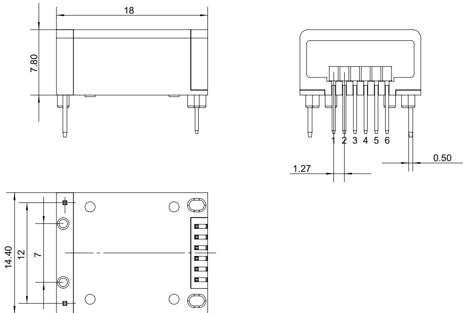
图 12 外形尺寸图 (尺寸单位: mm)
