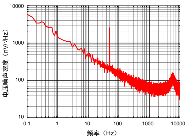
图 9 典型电压噪声谱密度曲线
