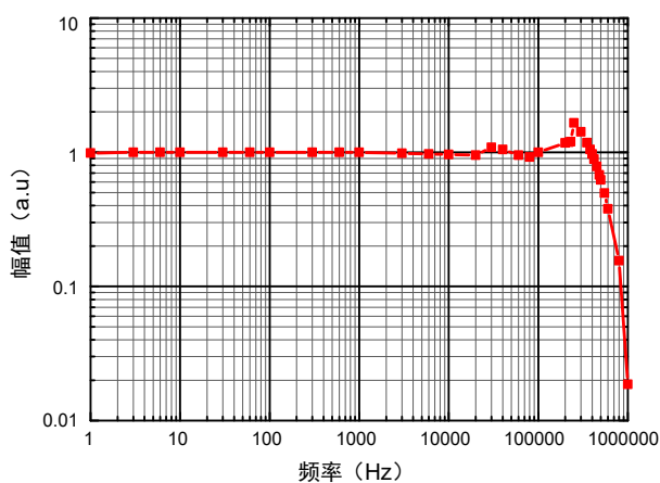
图 8 典型频率响应特性
