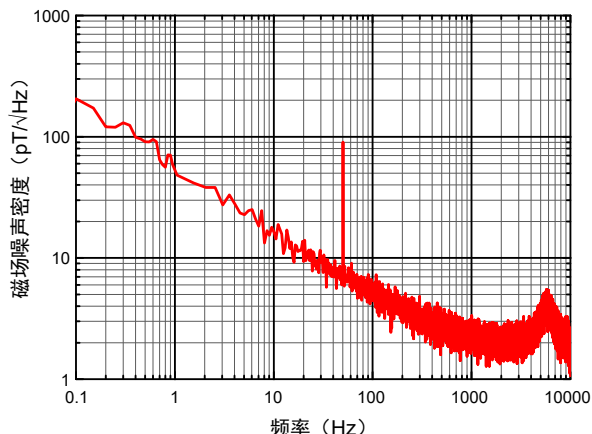
图 10 典型等效磁场噪声谱密度曲线
