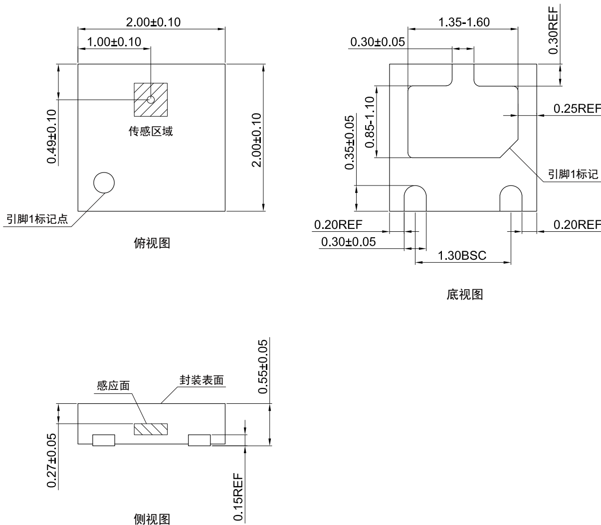
图 7 DFN3L (2×2×0.55) 封装图 (尺寸单位: mm)
