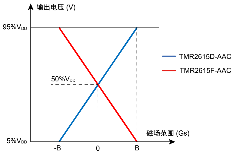
图 5 电压输出曲线
