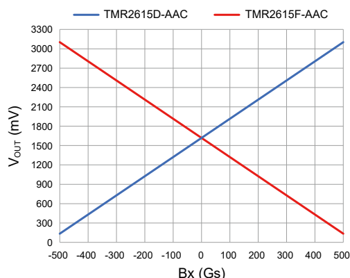
TMR2615x-AAC \pm 500 Gs 输出曲线
