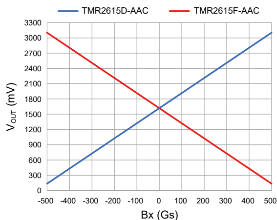
图 3 TMR2615x-AAC 芯片输出曲线
