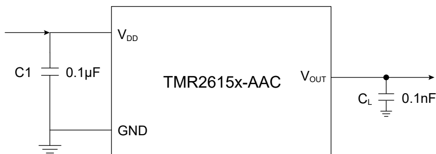
图 6 应用电路图
