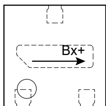
图 2-3 芯片轴向图 (DFN3L(1.6×1.6) 俯视图)
