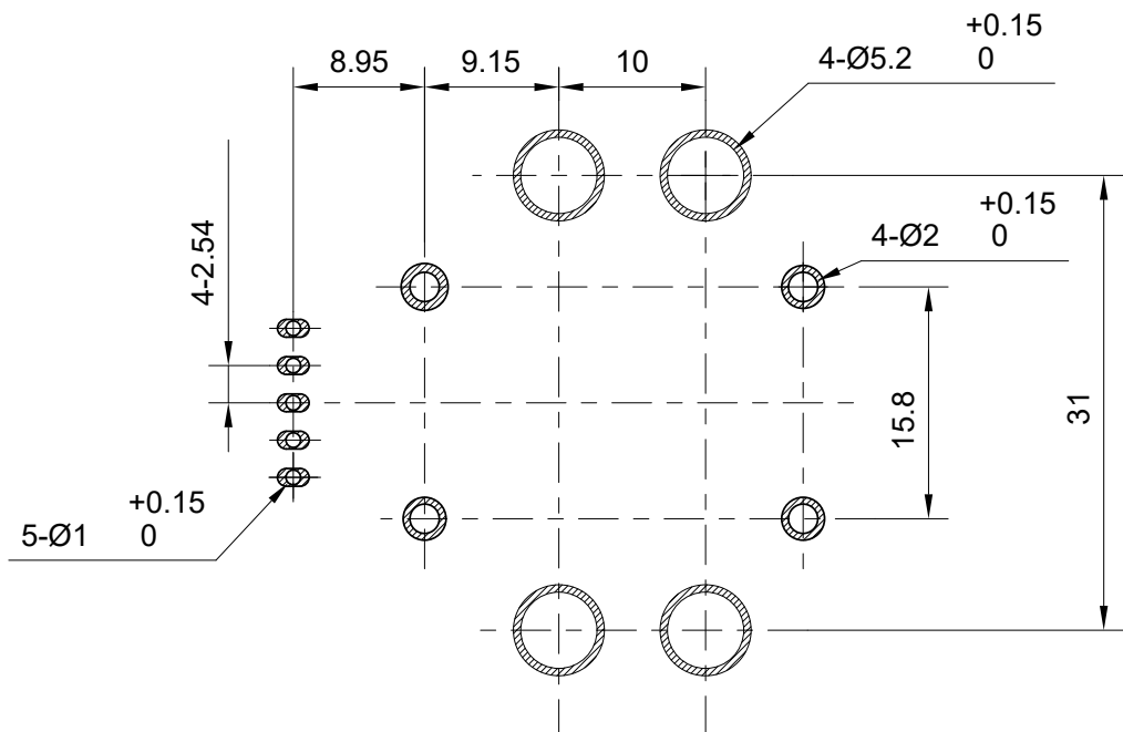
图 14 推荐焊盘示意图（尺寸单位：mm）
