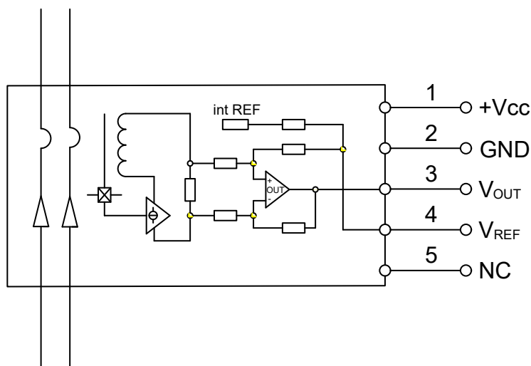
图 12 电气连接图
