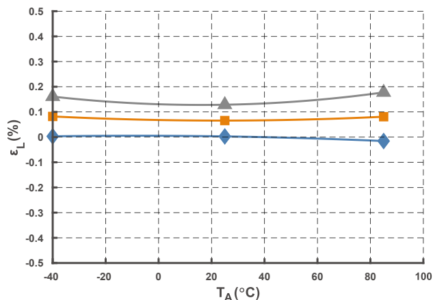
图 8 线性度曲线
