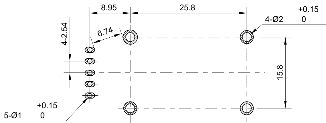
图 15 推荐焊盘示意图（尺寸单位：mm）
