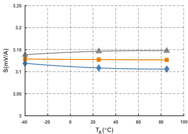
图 11 灵敏度曲线
