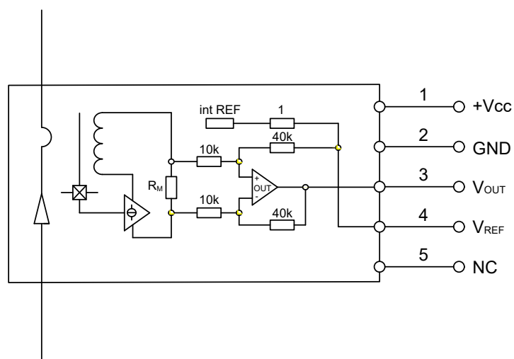
图 13 电气连接图
