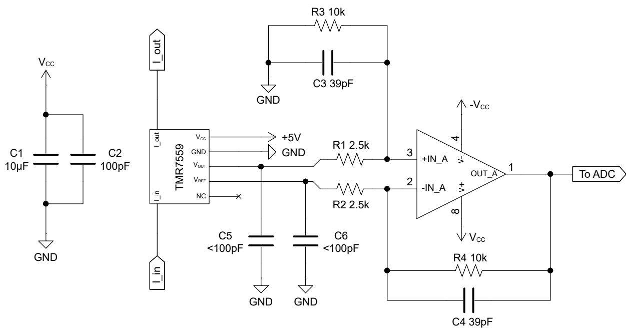
图 16 典型应用电路图
