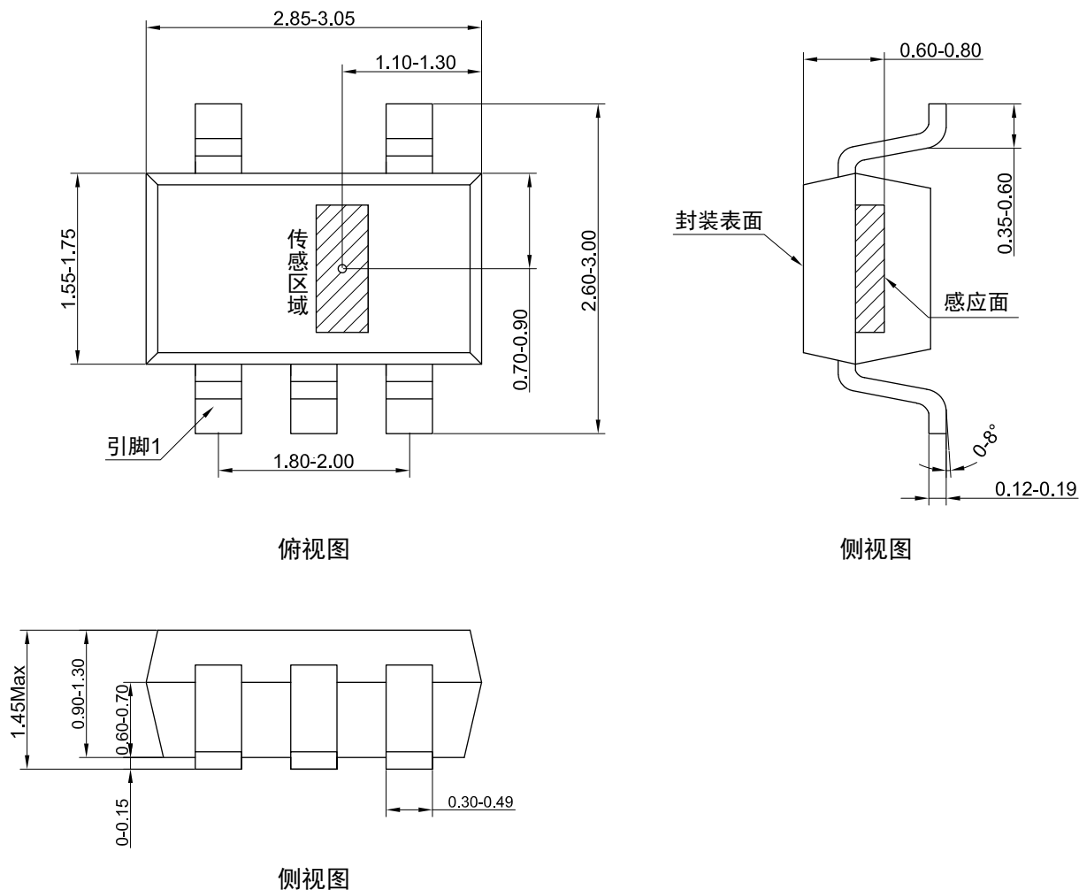
图 4 SOT23-5 封装图 (尺寸单位: mm)
