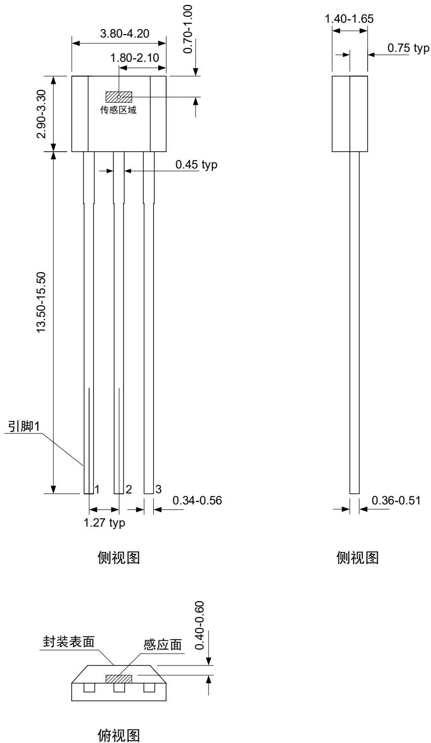
图 9 TO92S 封装图 (尺寸单位: mm)
