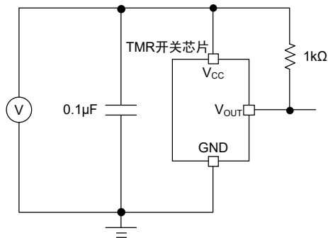
图 7 滤波电容用以降低供电噪音
