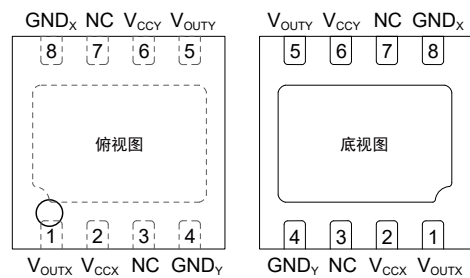
图 4 引脚定义
