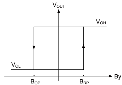
图 3-2 芯片磁场响应曲线
