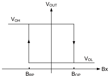
图 3-1 芯片磁场响应曲线
