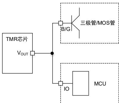
图 14 驱动功率负载的应用电路
