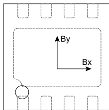
图 2-2 芯片敏感轴向图 (DFN8L 俯视图)
