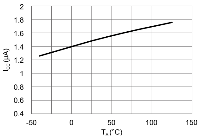
图 13 工作电流和工作温度的关系 (V CC = 3 V)
