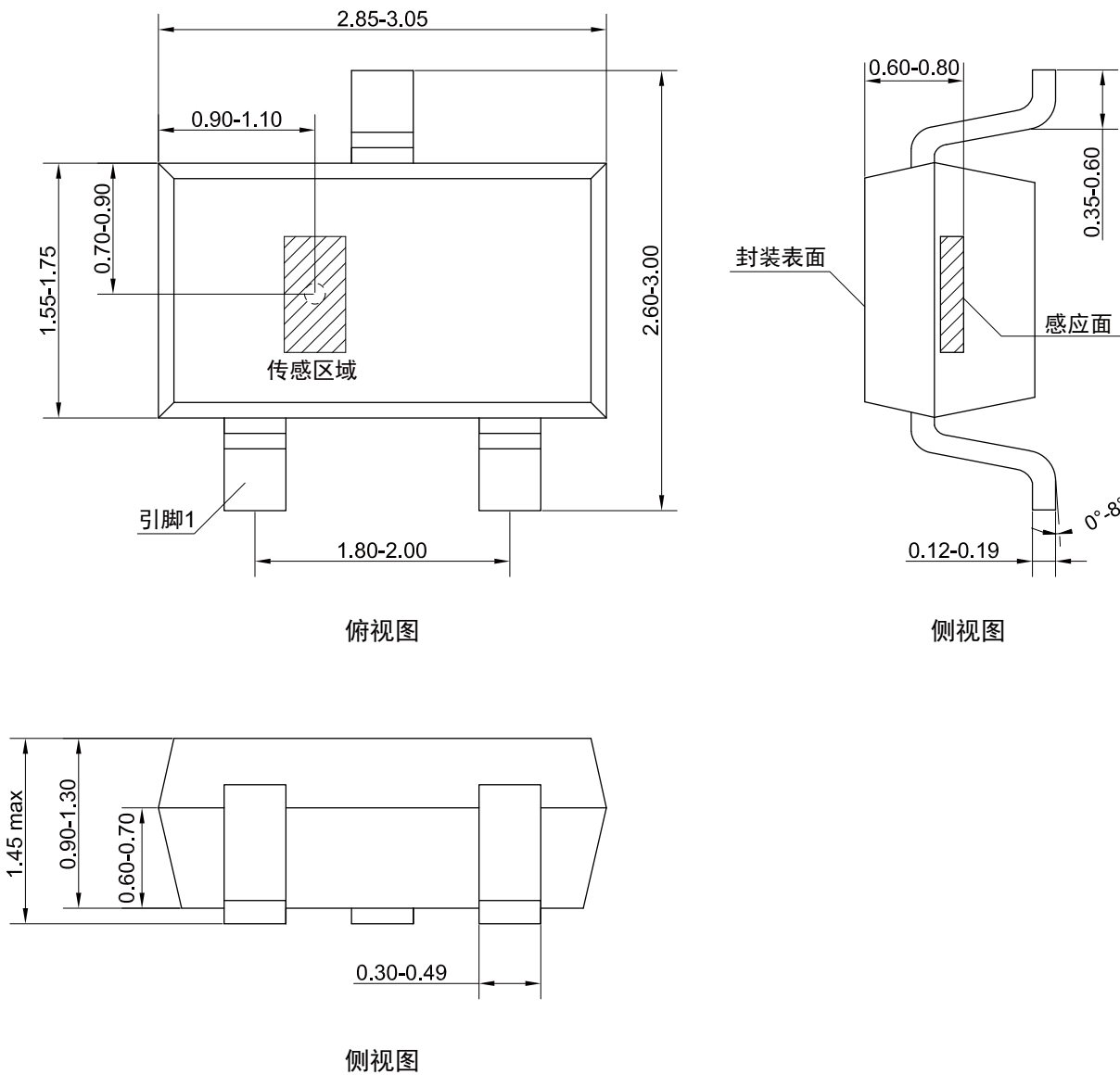
图 25 SOT23-3 封装图 (尺寸单位: mm)
