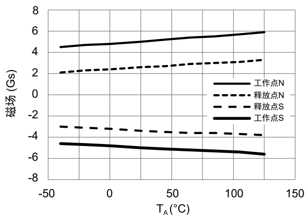
图 22 工作点、释放点和工作温度的关系 (V CC = 3 V)
