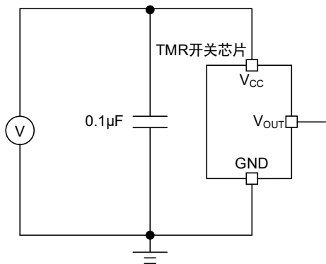
图 23 滤波电容用以降低供电噪音
