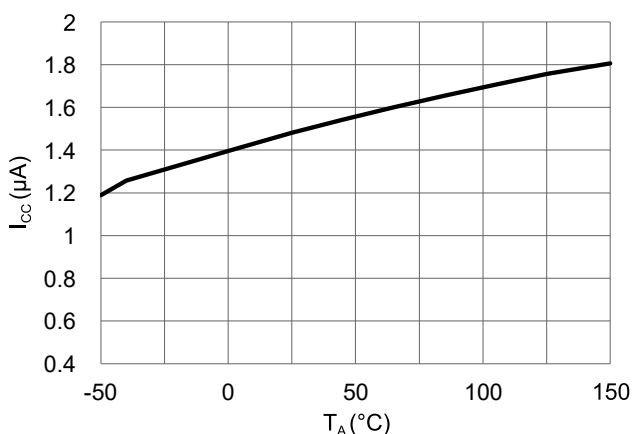
图 15 工作电流和工作温度的关系 (V CC = 3 V)
