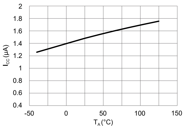
图 17 工作电流和工作温度的关系 (V CC = 3 V)
