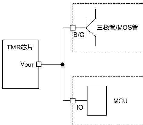
图 24 驱动功率负载的应用电路
