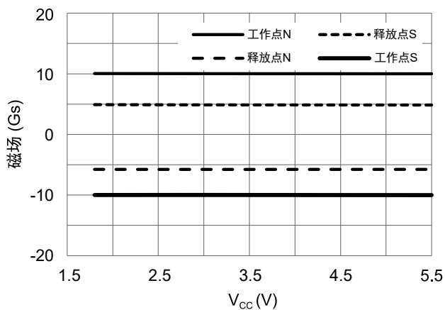
图 10 工作点、释放点和供电电压的关系 (T A = 25 °C)
