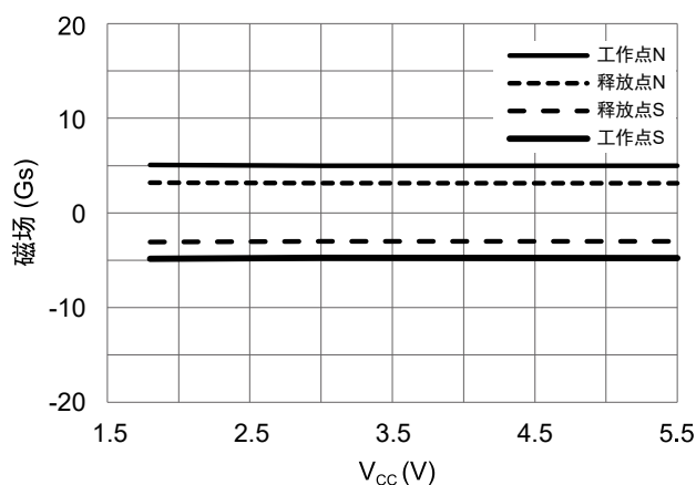
图 12 工作点、释放点和供电电压的关系 (T A = 25 °C)
