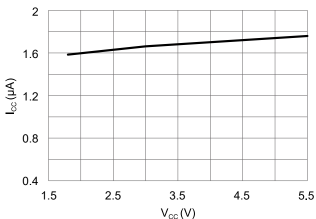
图 11 工作电流和供电电压的关系 (T A = 25 °C)
