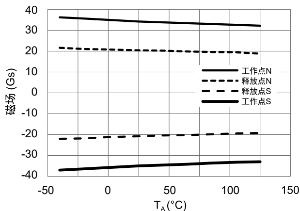
图 18 工作点、释放点和工作温度的关系 (V CC = 3 V)
