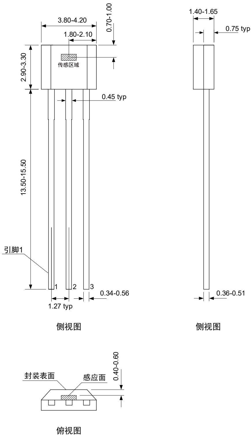
图 26 TO92S 封装图 (尺寸单位: mm)
