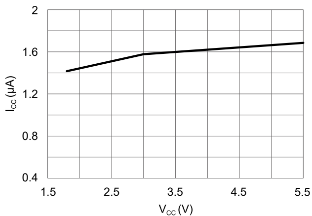
图 9 工作电流和供电电压的关系 (T A = 25 °C)
