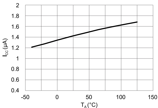
图 19 工作电流和工作温度的关系 (V CC = 3 V)
