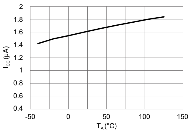
图 21 工作电流和工作温度的关系 (V CC = 3 V)
