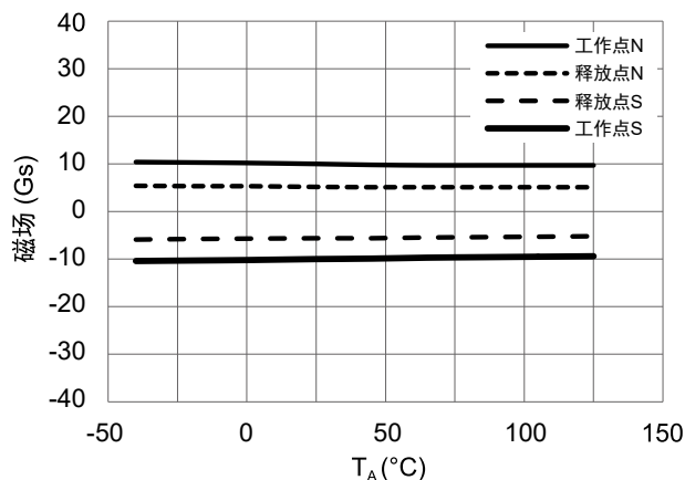
图 20 工作点、释放点和工作温度的关系 (V CC = 3 V)
