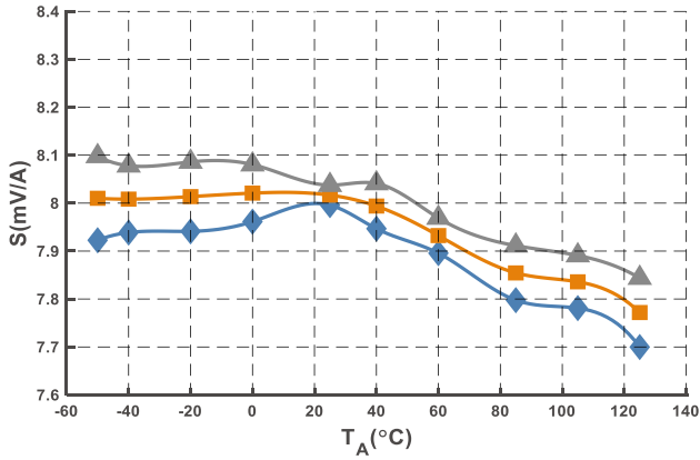
图 12 灵敏度曲线 (@I PN = 500 A)
