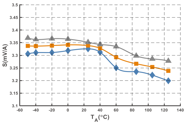
图 16 灵敏度曲线 (@I PN = 1200 A)
