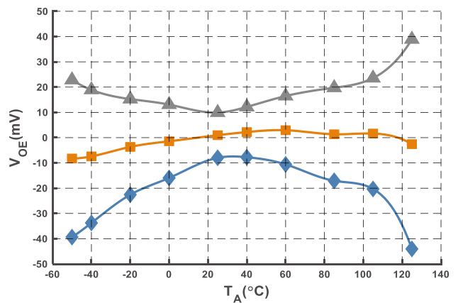
图9 零点失调电压曲线
