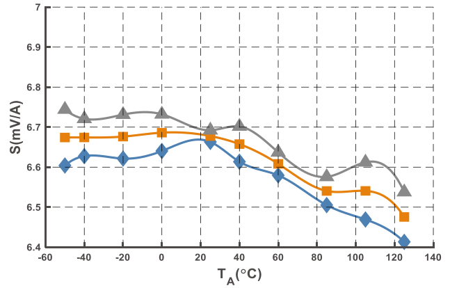
图 13 灵敏度曲线 (@I PN = 600 A)
