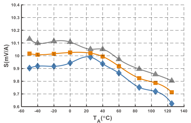
图11 灵敏度曲线 (@I PN = 400 A)
