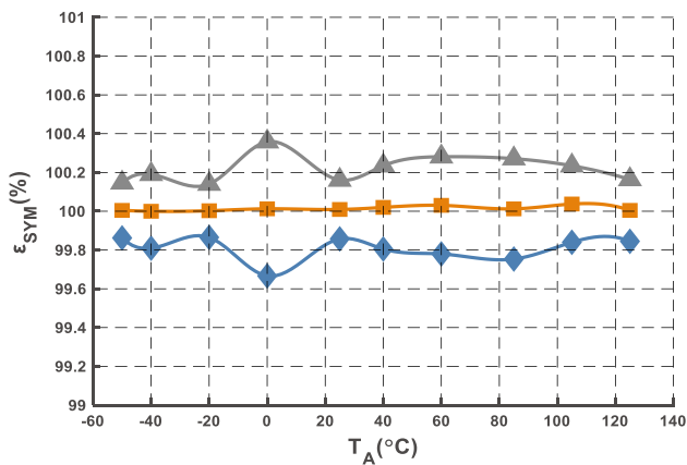
图8 增益对称性曲线
