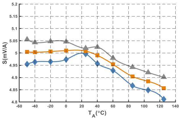
图 14 灵敏度曲线 (@I PN = 800 A)
