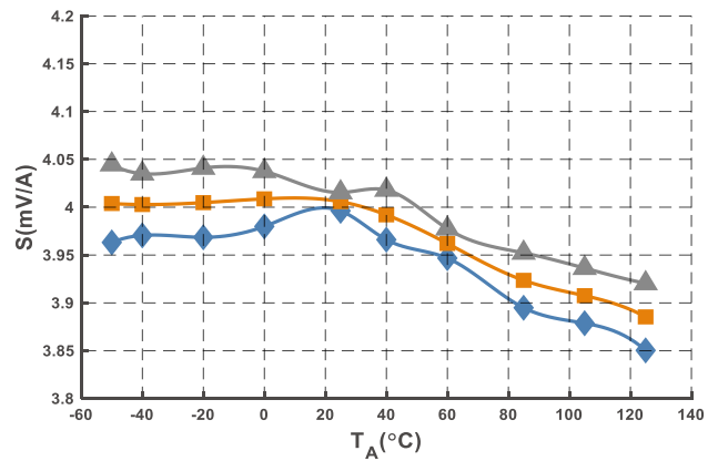
图 15 灵敏度曲线 (@I PN = 1000 A)
