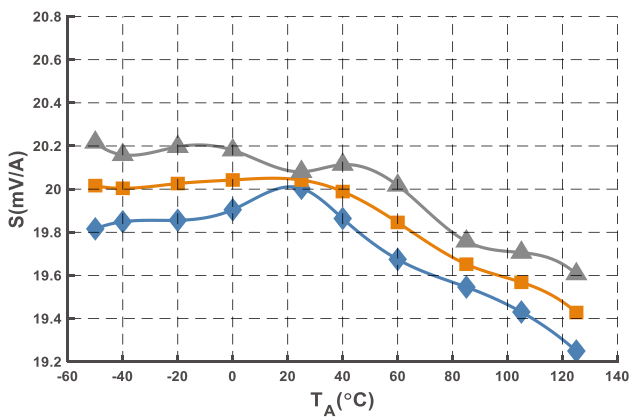
图10 灵敏度曲线 (@I PN = 200 A)
