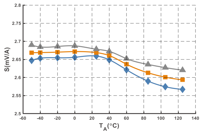
图 17 灵敏度曲线 (@I PN = 1500 A)
