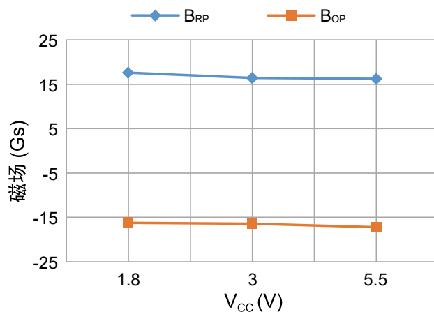
图 5 工作点、释放点和供电电压的关系 ( T_A = 25\text{ °C} )
