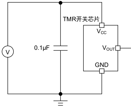
图 7 滤波电容用以降低供电噪音
