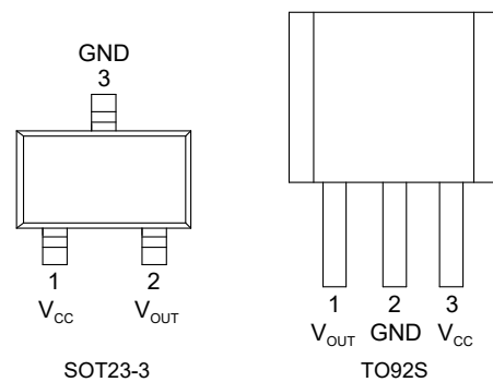
图 4 引脚定义
