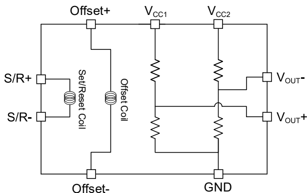
图 1 芯片内部原理框图
